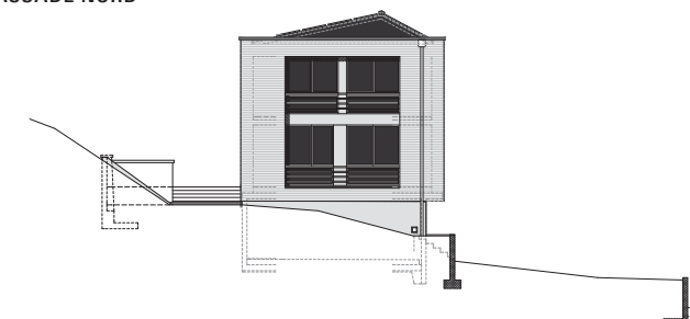
FASSADE NORD
