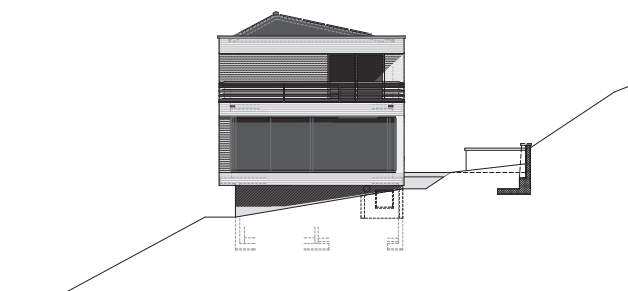
FASSADE SÜD
